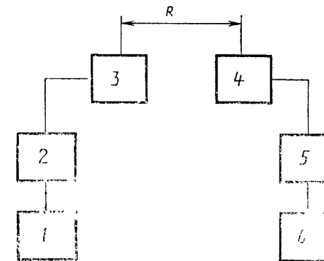
1 — генератор; 2 — аттенюатор; 3 — передающая антенна; 4 — приемная антенна; 5 — аттенюатор; 6 — измерительный приемник
